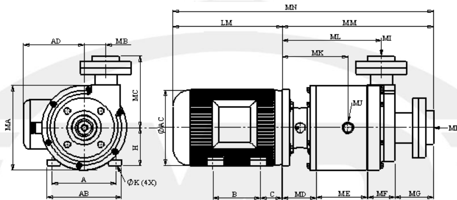
Figura. Bomba Master BSD 10-40/ BSD 10-45
