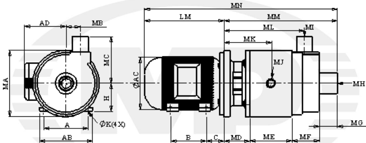
Figura. Bomba Master B de 0,5-1,5CV
